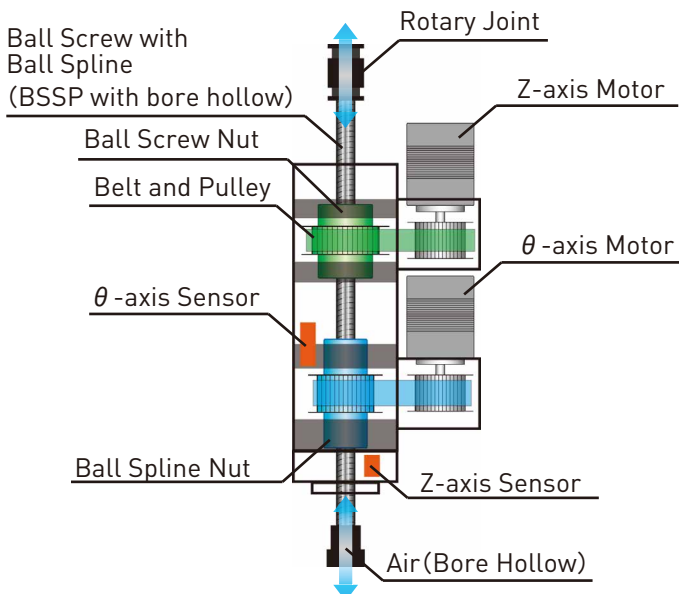
【Belt Drive】
